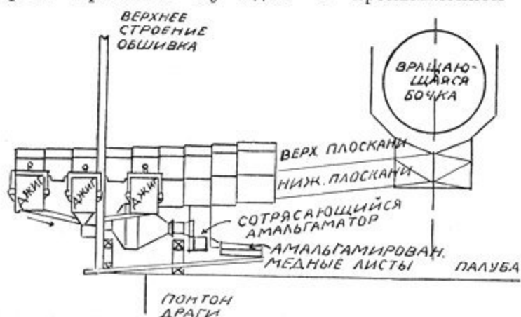
Черт. 20. Попер. разрез, показ. установку джагов, мельницы Гардинга и Альмагаматора на Иосем. драге.
