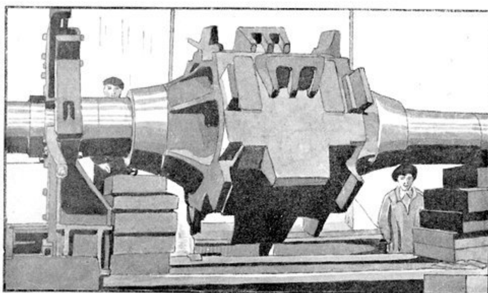
В. Целый верхний барабан, отлитый вместе с осью; драга Юба № 14.
