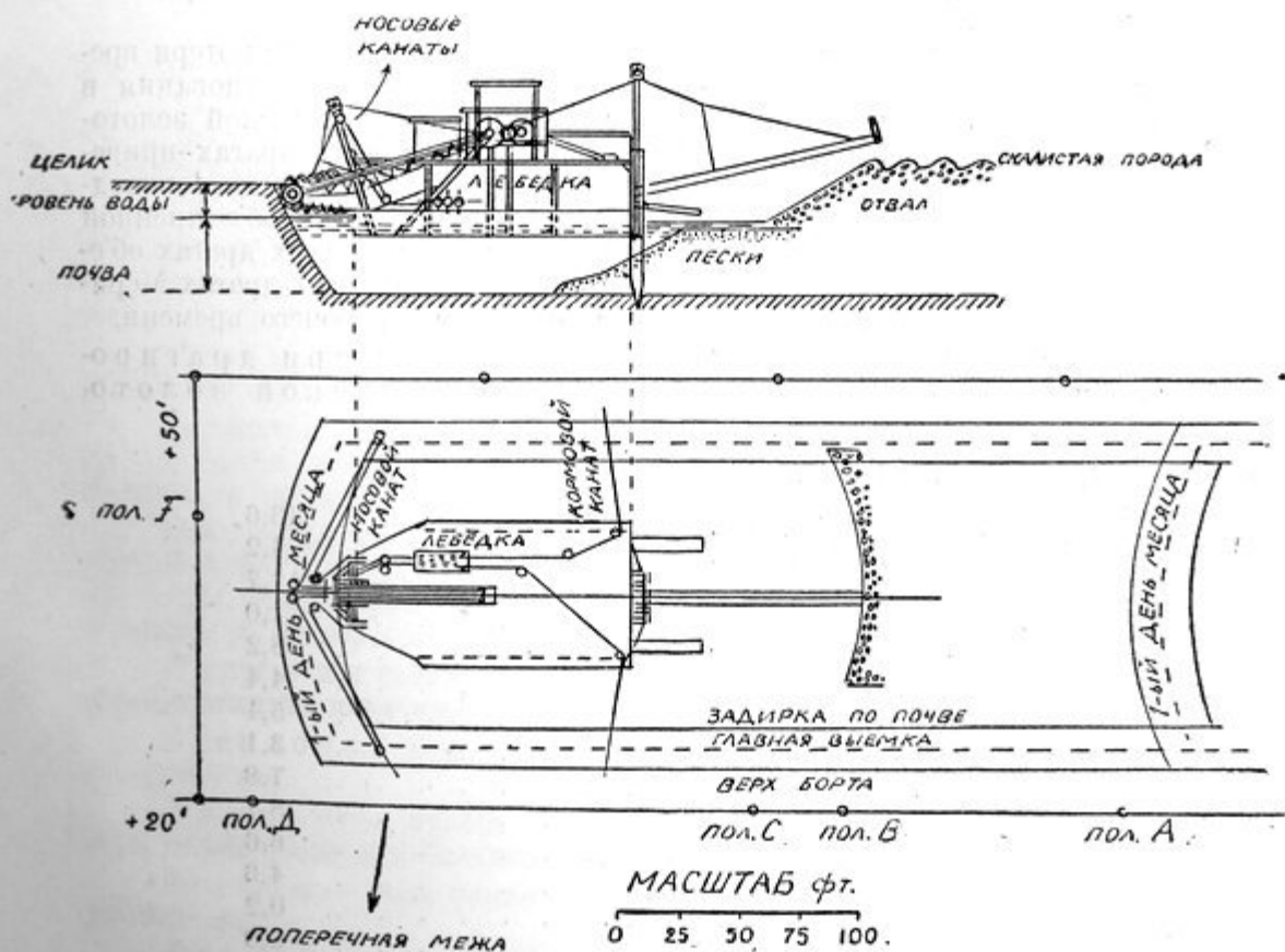
Чертеж 18: план и вертикальный продольный разрез 9' драги, показывающий лебедки и канаты для бокового передвижения драги, а также способы вычисления кубажа.
