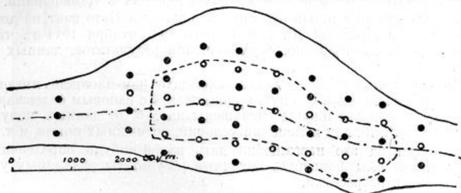
Чертеж 4: Расположение буровых скважин.
