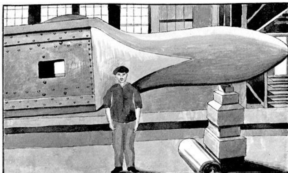
А. Круглый наконечник из литой стали для сваи.
