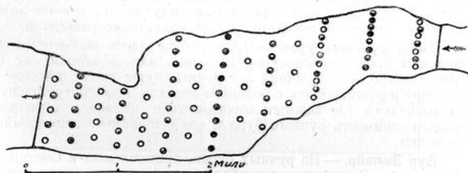
Чертеж 5: Расположение буровых скважин.
