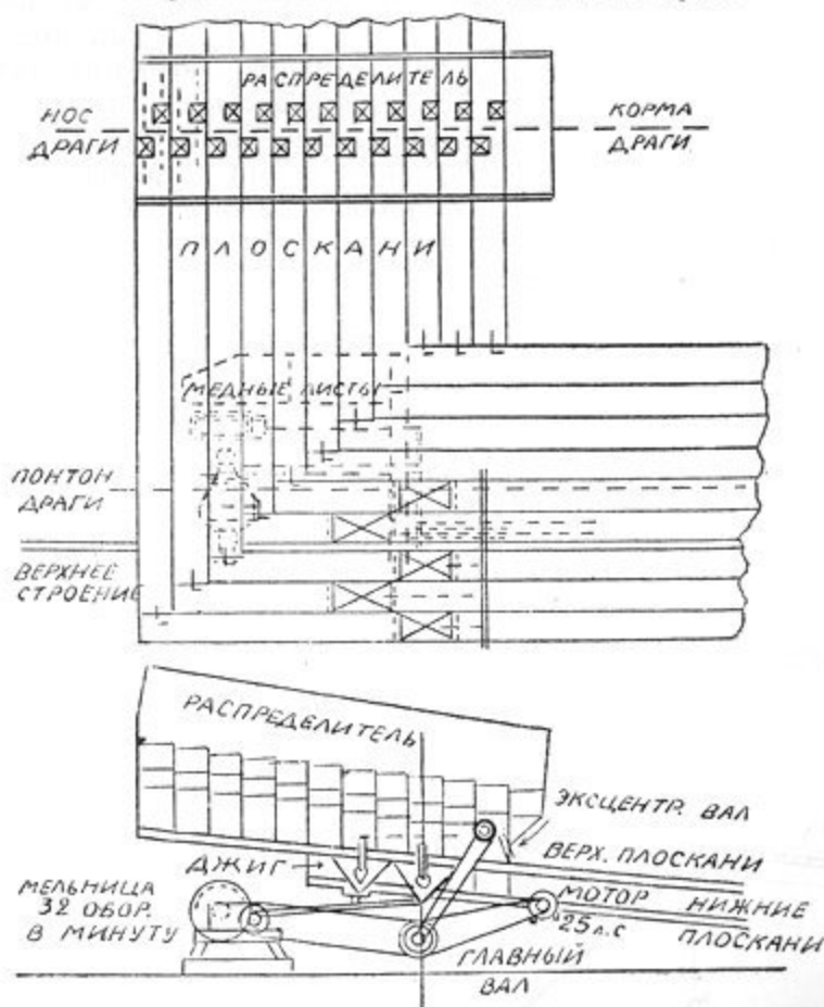
Черт. 21. План и разрез золотоулав. столов (посеканей), показ. расположение и приводы для джагов и мельницы.
