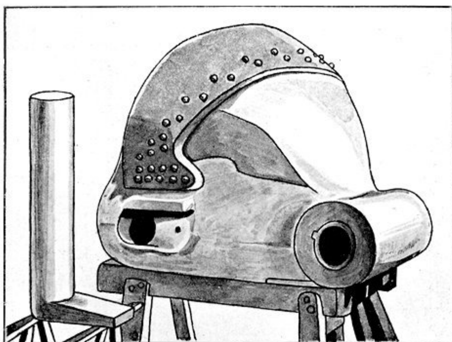
С. Ковш из марганцевистой стали, объемом в 16 куб. фут. драги Конрей № 4; в заднее ухо вставлена цельная цилиндрическая втулка.
