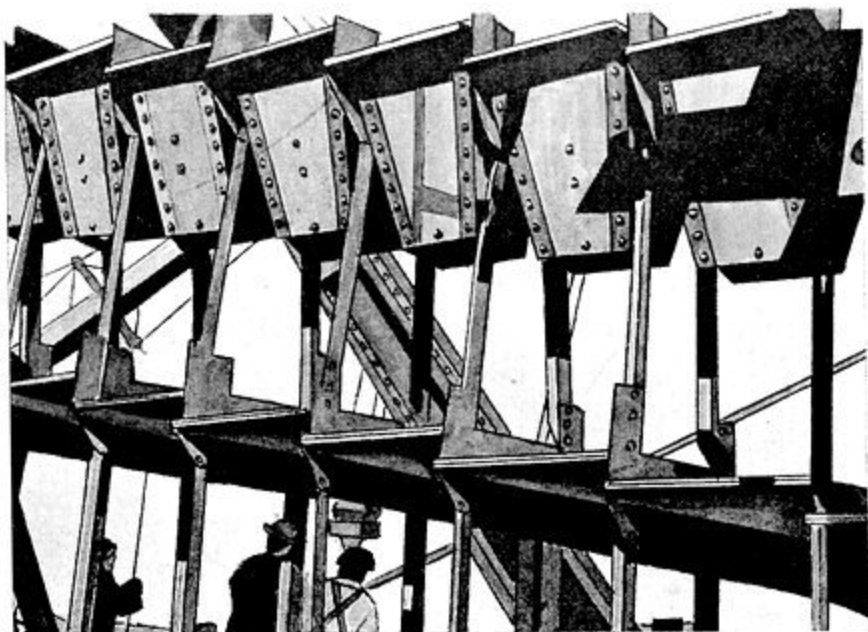
А. Боковой вид распределителя на драге Юба. Плоскани (столы) не установлены.
