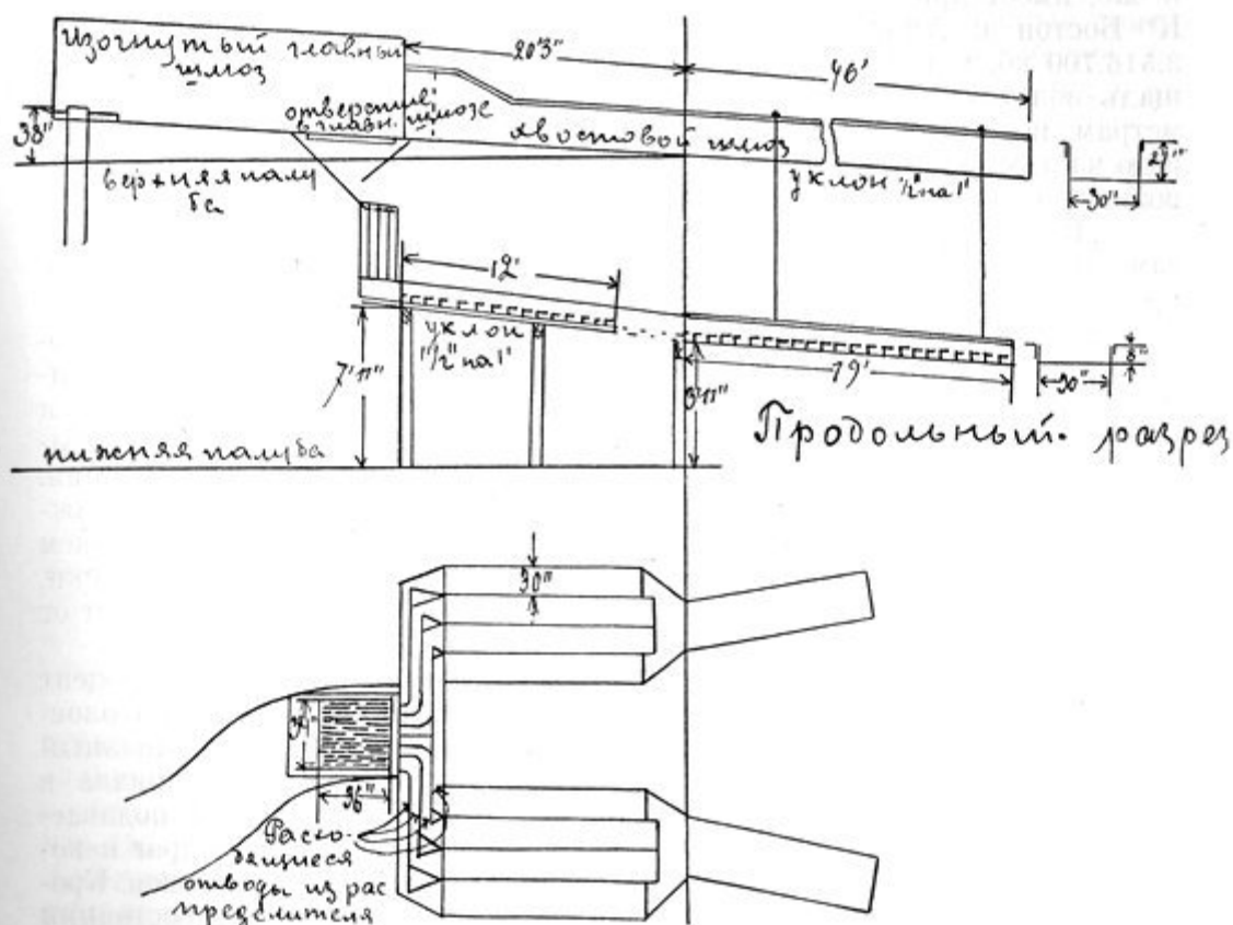
Черт. 22. План и разрез системы подставных шлюзов, примен. на драге № 3 в Брекенридже. Колорадо.
